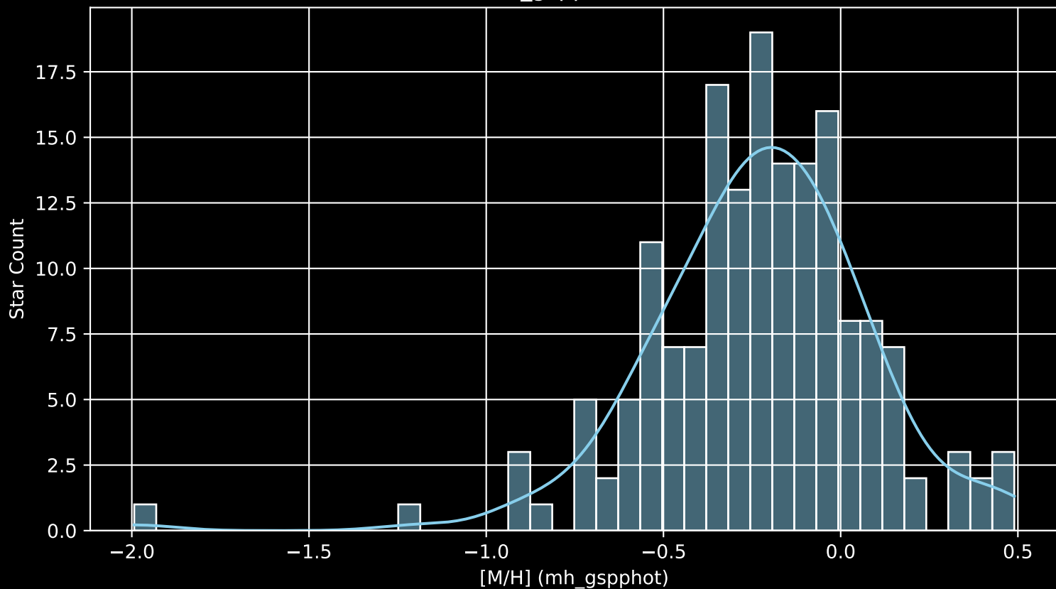
APOGEE DR17 Field: [280-27 [M/H] (mh_gspphot) (n= 169)
