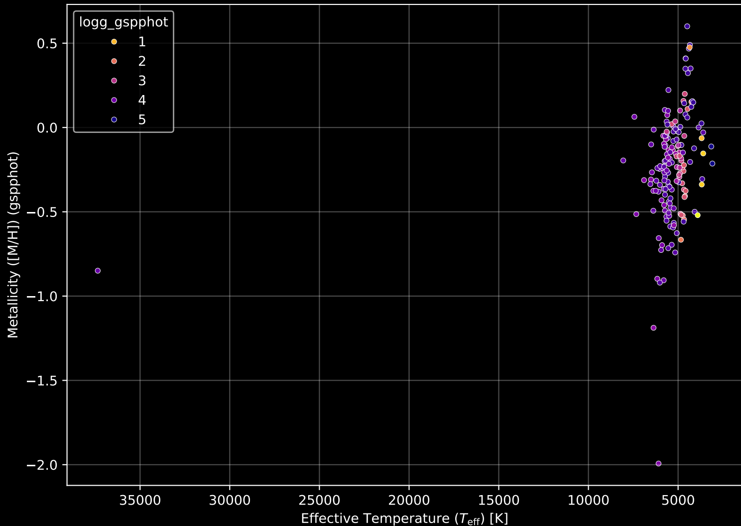
APOGEE DR17 Field: [280-27] Stellar Population Parameters (n= 170)
