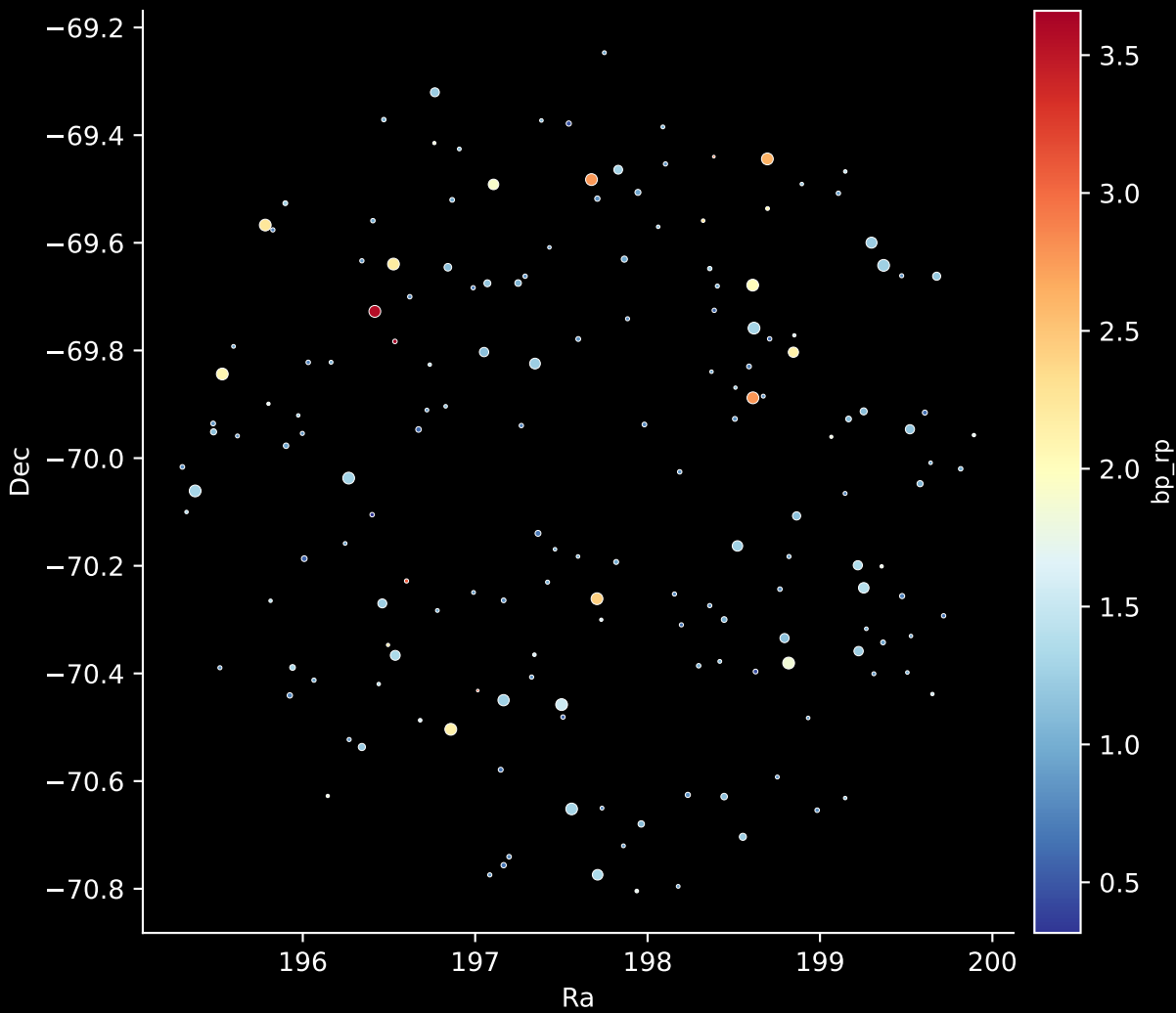
APOGEE DR17 Field: [280-27] Stars: 170
